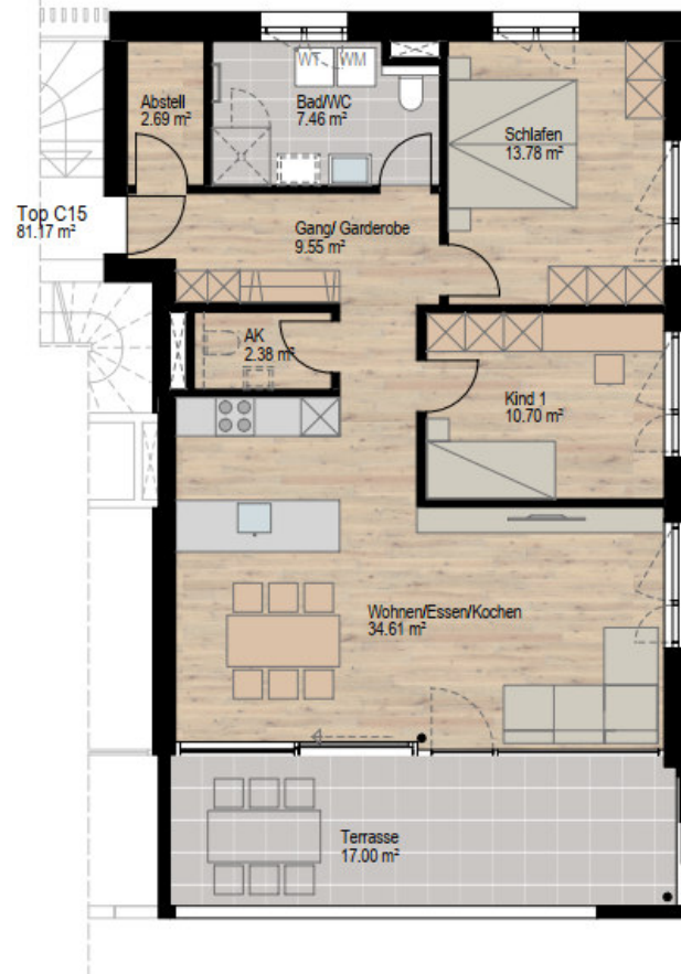
Variante 3-Zi-Wohnung
