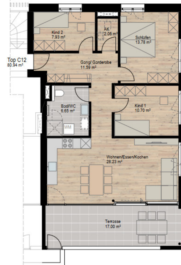
Variante 4-Zi-Wohnung
