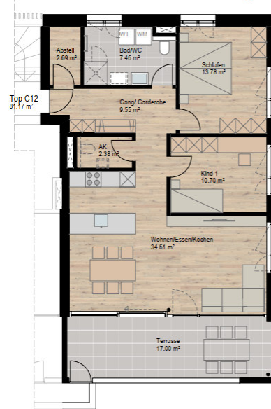
Variante 3-Zi-Wohnung
