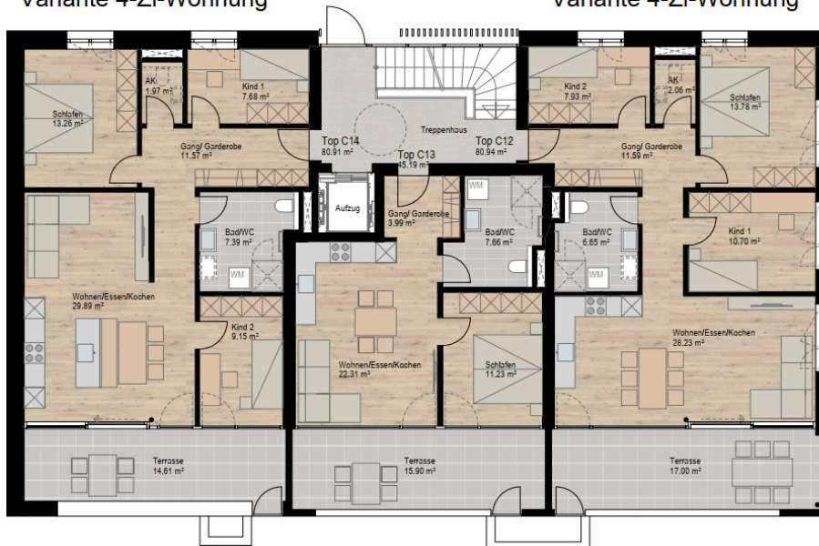
Variante 4-Zi-Wohnung
