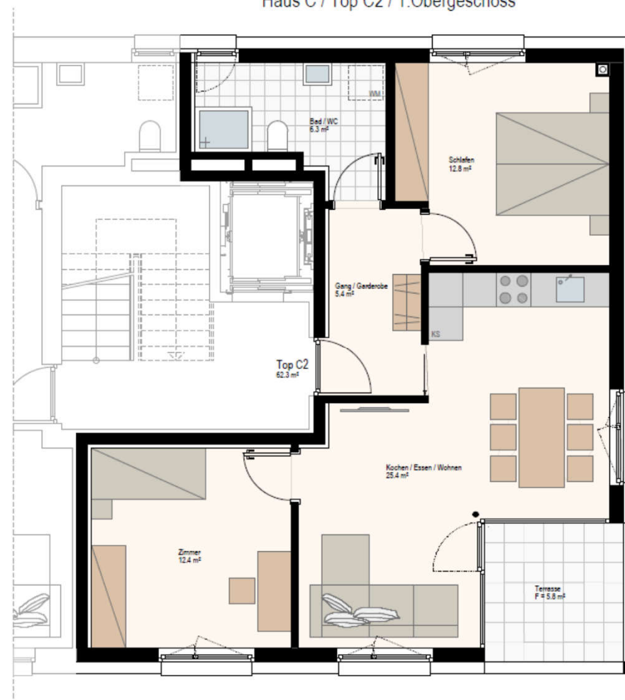
Haus C / Top C2 / 1.Obergeschoss
