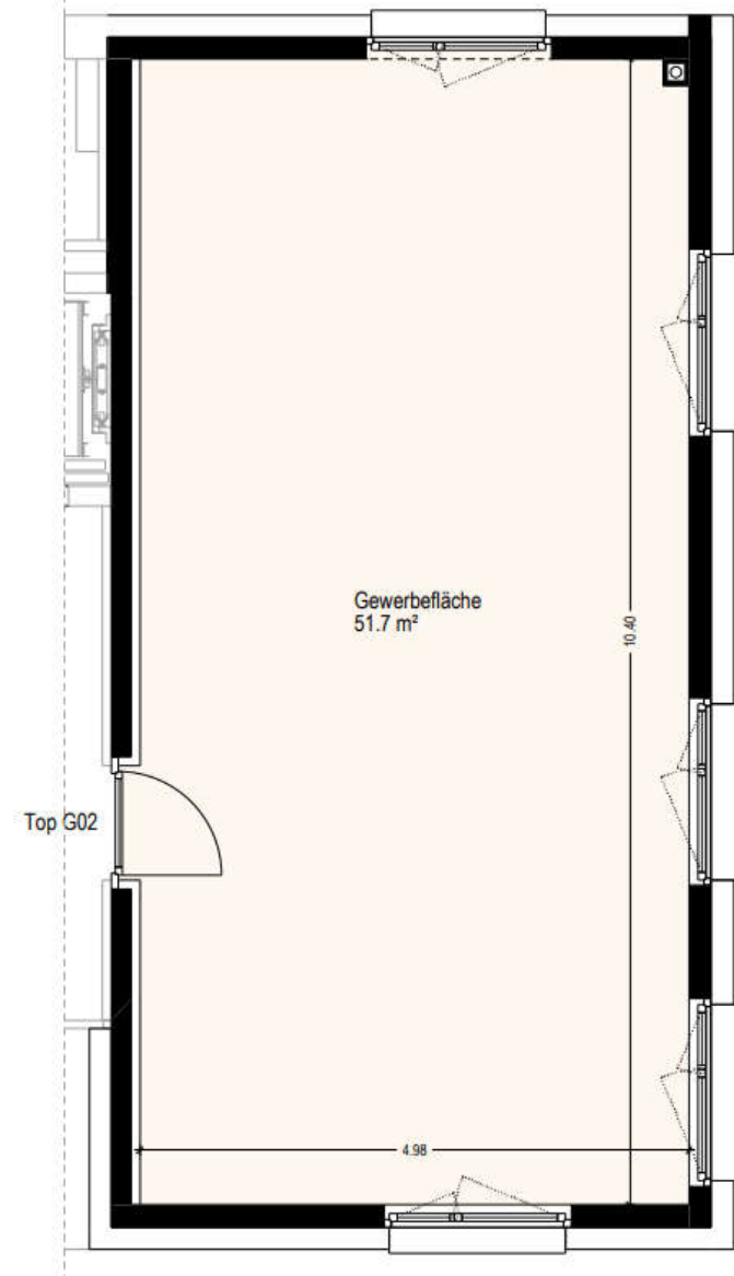
Haus C / Top G02 / Erdgeschoss
