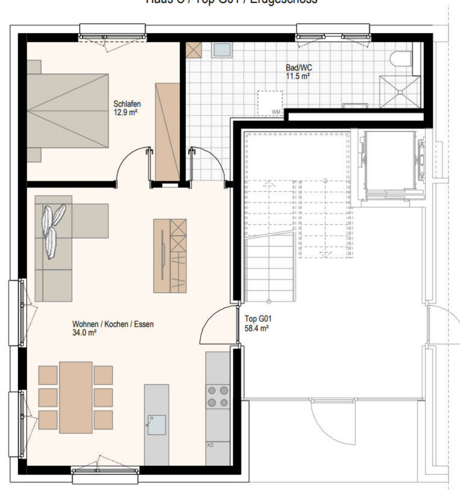
Haus C / Top G01 / Erdgeschoss
