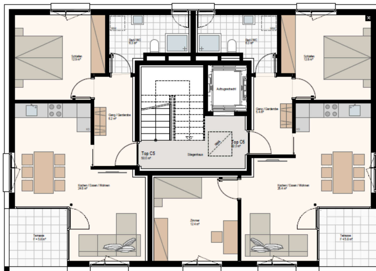
Haus C / 3.Obergeschoss
